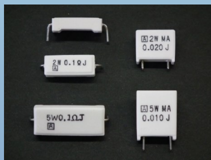
セメント抵抗
